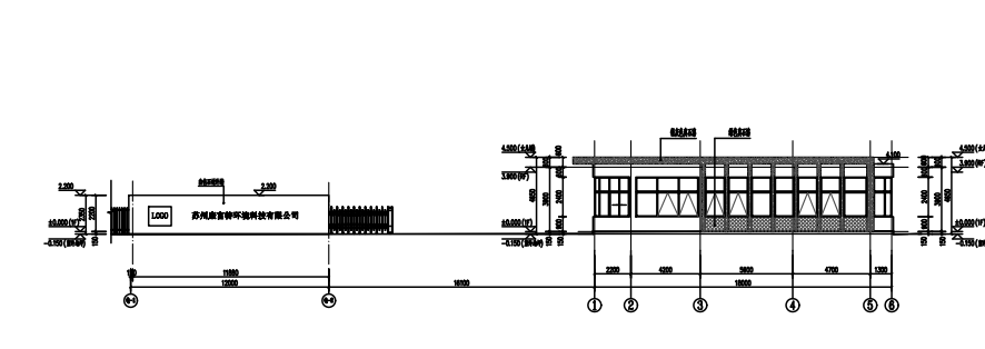
4#门卫 ①-⑥立面图
