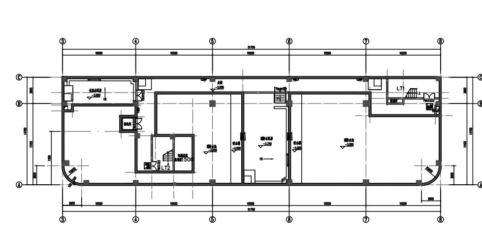
1#办公楼 地下一层平面图
