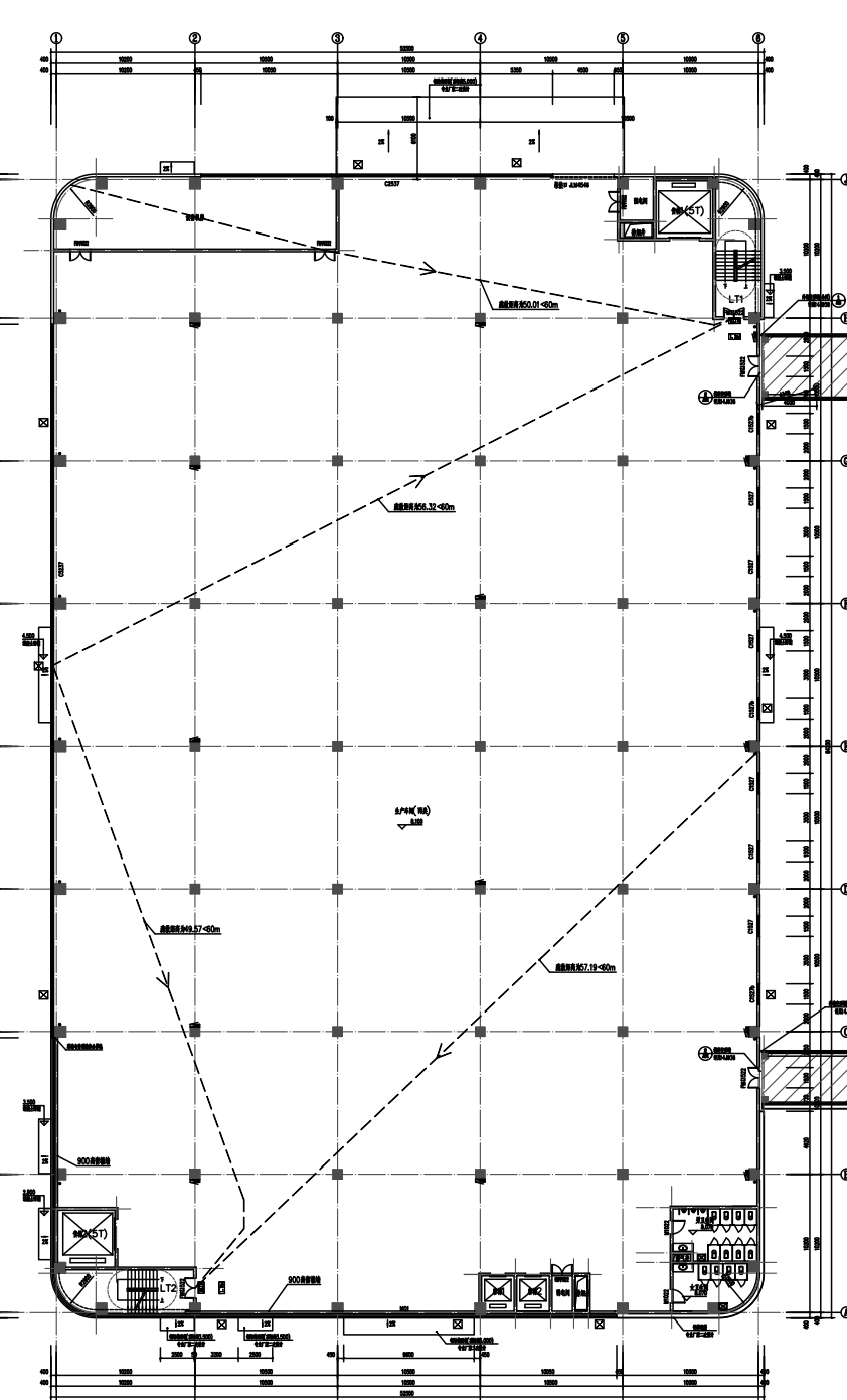
3#生产厂房 二层平面图
