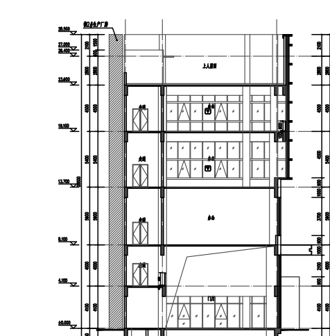
1#办公楼 1-1剖面图
