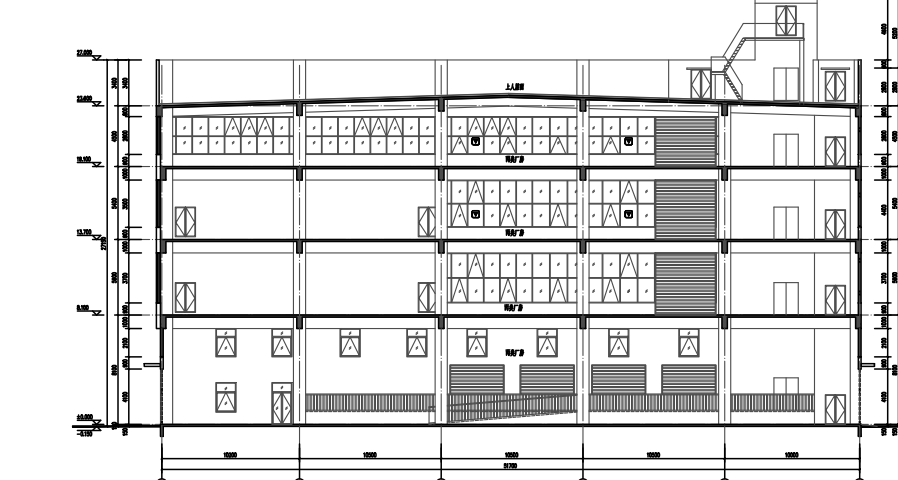
3#生产厂房 1-1剖面图
