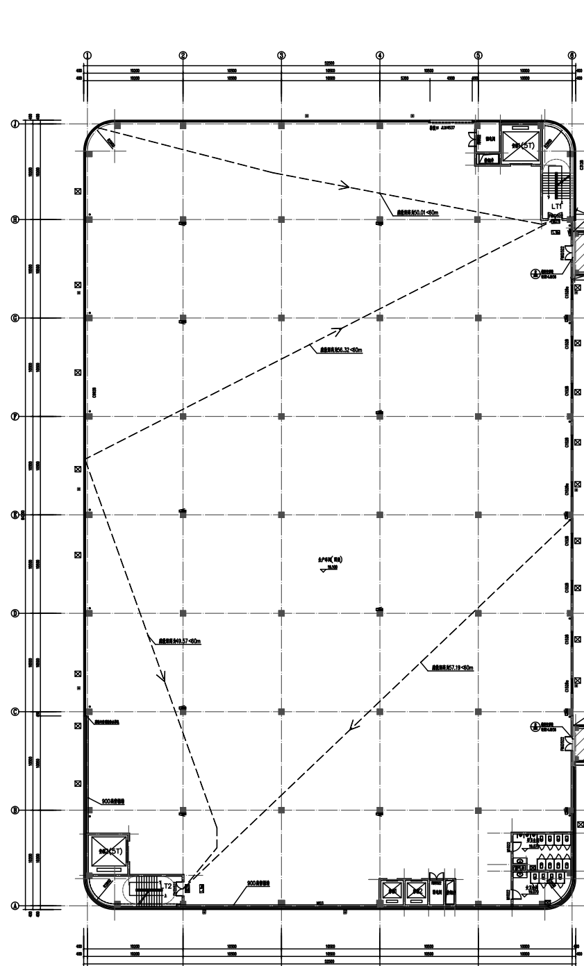
3#生产厂房 四层平面图
