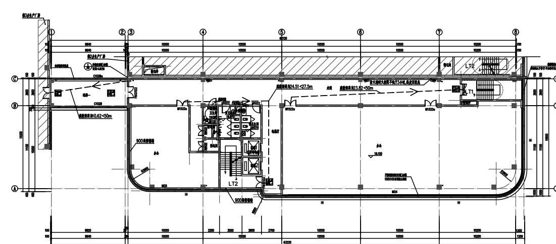
1#办公楼 一层平面图
