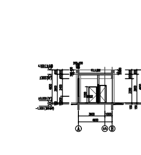
4#门卫 1-1剖面图
