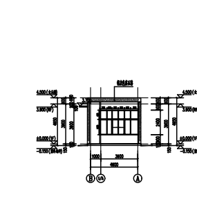
4#门卫 B-A立面图
