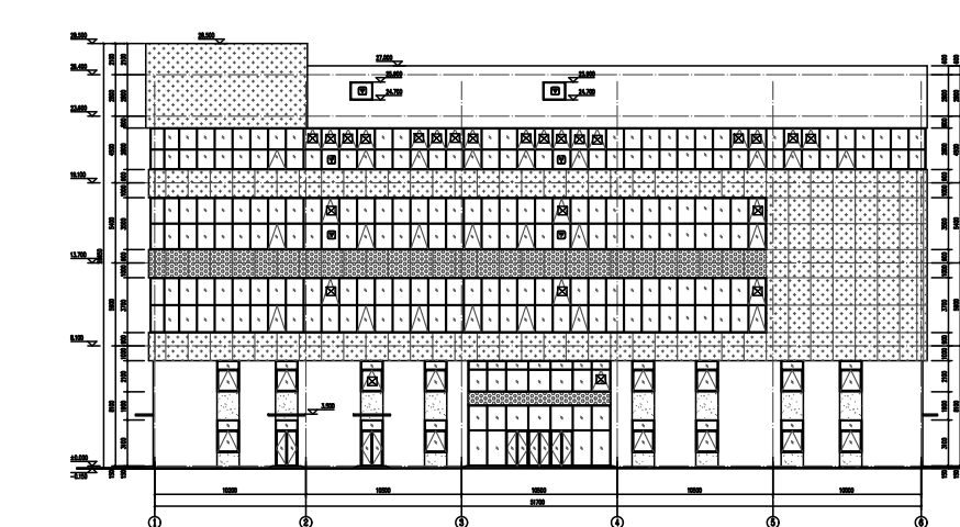
3#生产厂房 ①-⑥立面图
