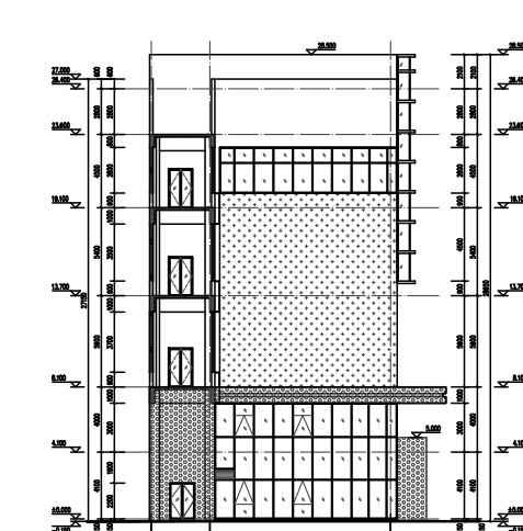
1#办公楼 ⑧-A立面图
