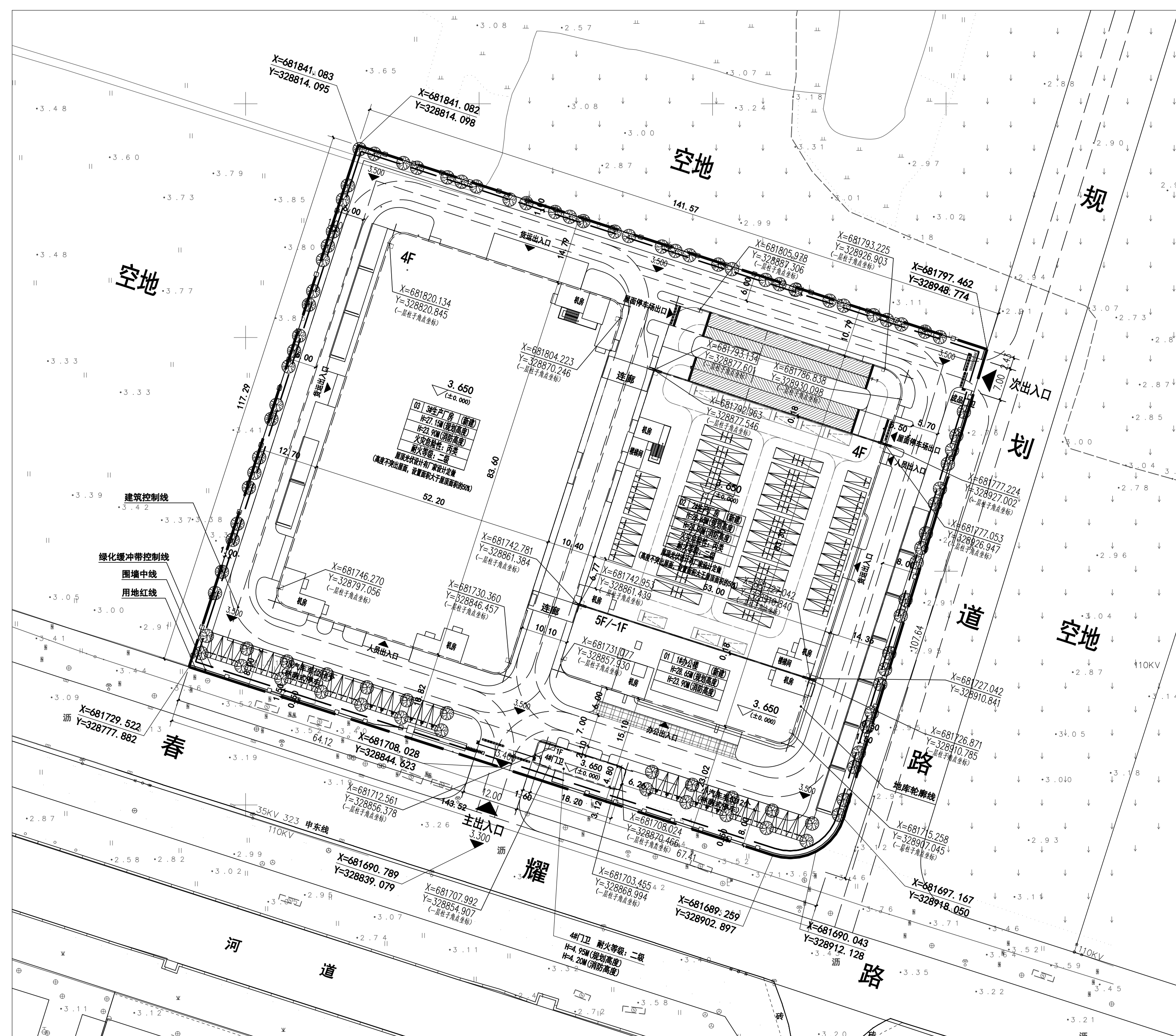
总平面图
