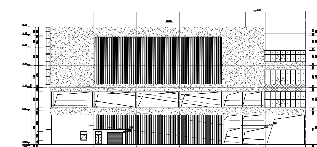
2#生产厂房 ⑧-①立面图
