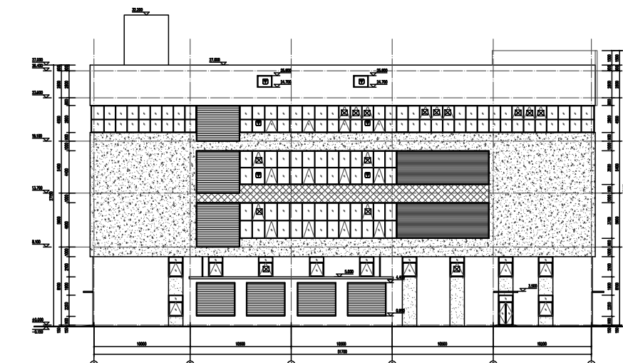
3#生产厂房 ⑥-①立面图
