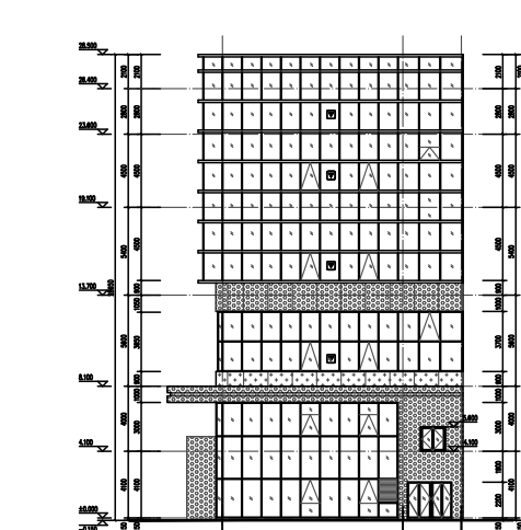
1#办公楼 A-⑥立面图
