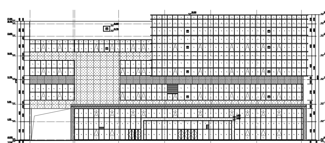
1#办公楼 ①-⑧立面图
