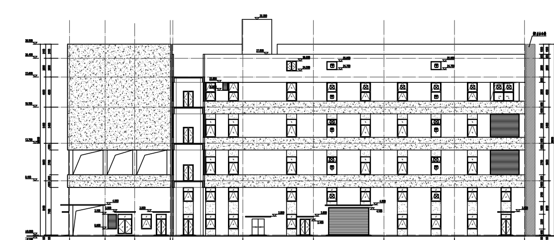
2#生产厂房 K-A立面图
