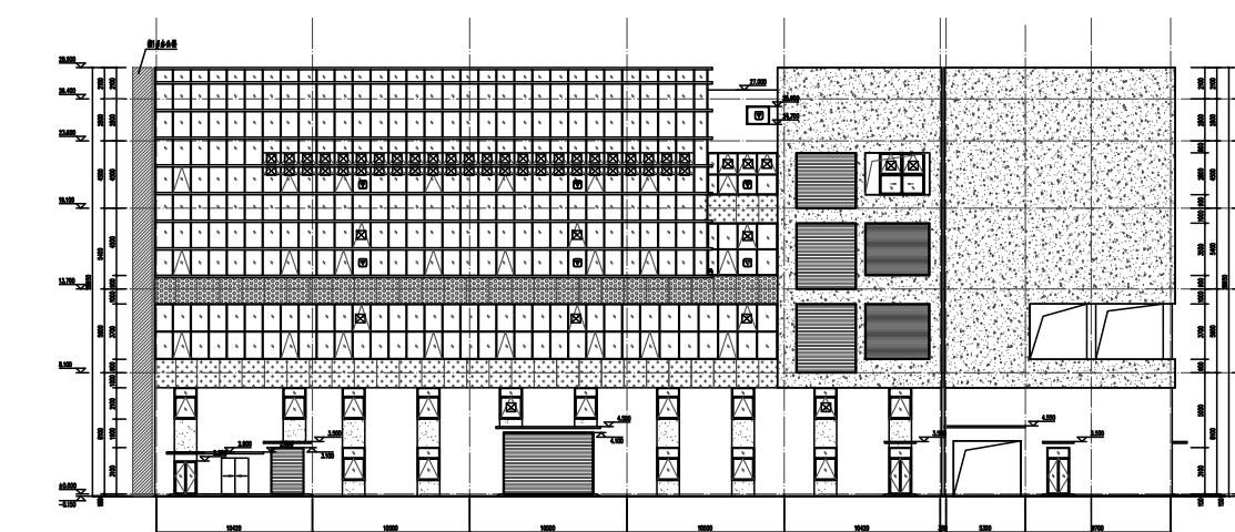
2#生产厂房 A-K立面图
