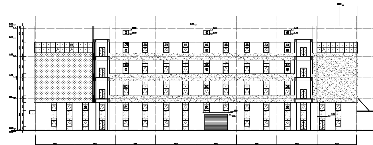
3#生产厂房 A-J立面图
